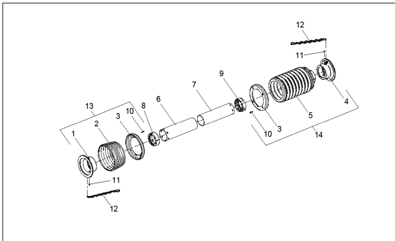
Rys. 32 ELEMENTY SKŁADOWE OSŁONY
