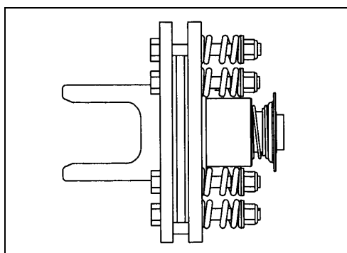
Rys. 31 SZKIC PRZEDSTAWIAJĄCY SPRZĘGŁO CIERNE-JEDNOKIERUNKOWE
