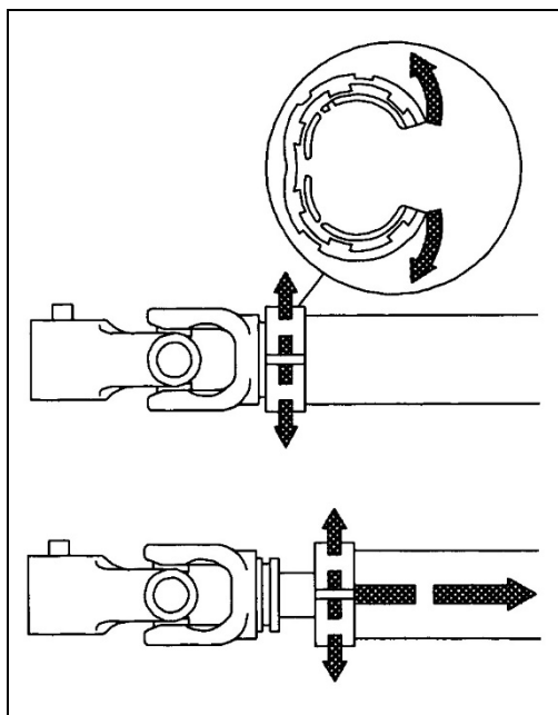
Rys. 20 ZSUNIECIE PIERŚCIENIA ŚLIZGOWEGO WRAZ Z RURĄ OSŁONY
