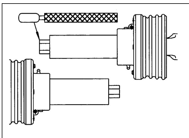
Rys. 14 SCHEMAT POKAZUJĄCY KRAWĘDZIE RUR, KTÓRE NALEŻY STĘPIĆ
