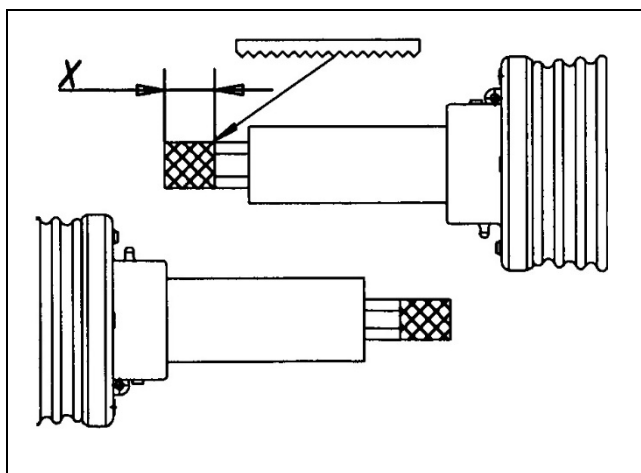
Rys. 13 SCHEMAT POKAZUJĄCY SPOSÓB SKRACANIA RUR TELESKOPU
