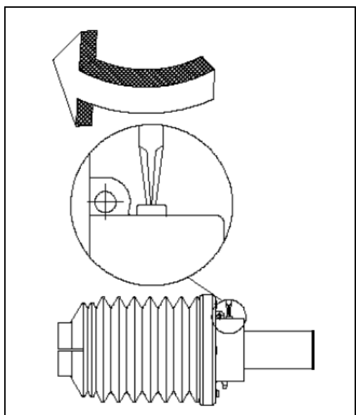
Rys. 26 WKRĘT MOCUJĄCY STOŻEK OSŁONY
