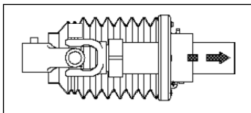
Rys. 19 ZSUNIĘCIE STOŻKA OSŁONY
