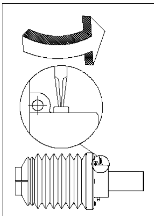
Rys. 17 WKRĘT MOCUJĄCY STOŻEK OSŁONY
