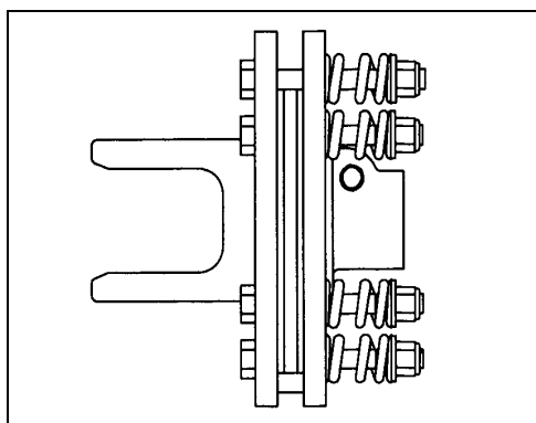
Rys. 28 SZKIC PRZEDSTAWIAJĄCY SPRZĘGŁO CIERNE
