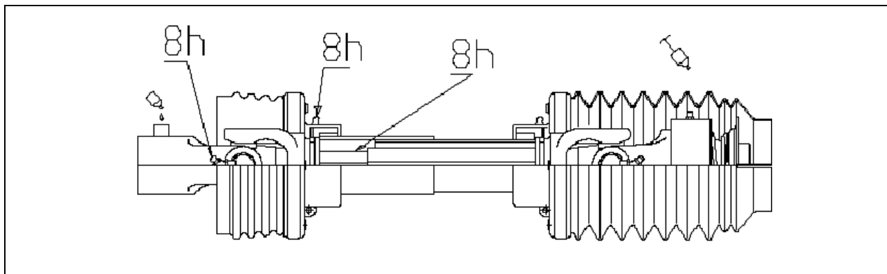
Rys. 11 SCHEMAT SMAROWANIA WAŁU PRZEGUBOWO-TELESKOPOWEGO
