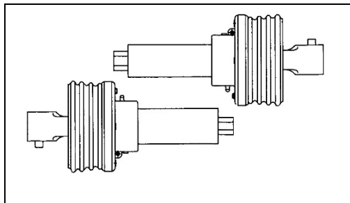
Rys. 16 DWIE CZĘŚCI WAŁU
