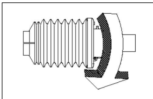
Rys. 18 OBRÓCENIE STOŻKA OSŁONY
